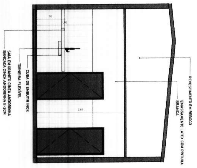
3 DETALHE BANCADA 1:25
